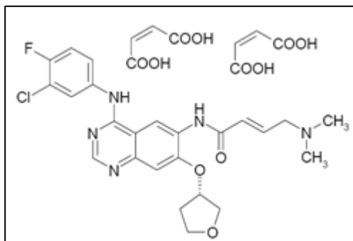
Abbildung 2: Chemische Struktur von Afatinib (N-[4-[(3-chloro-4-fluorophenyl)amino]-7-[[[(3S)-tetrahydro-3-furanyl]oxy]-6-quinazolinyl]-4-(dimethylamino)-2-butenamid])
