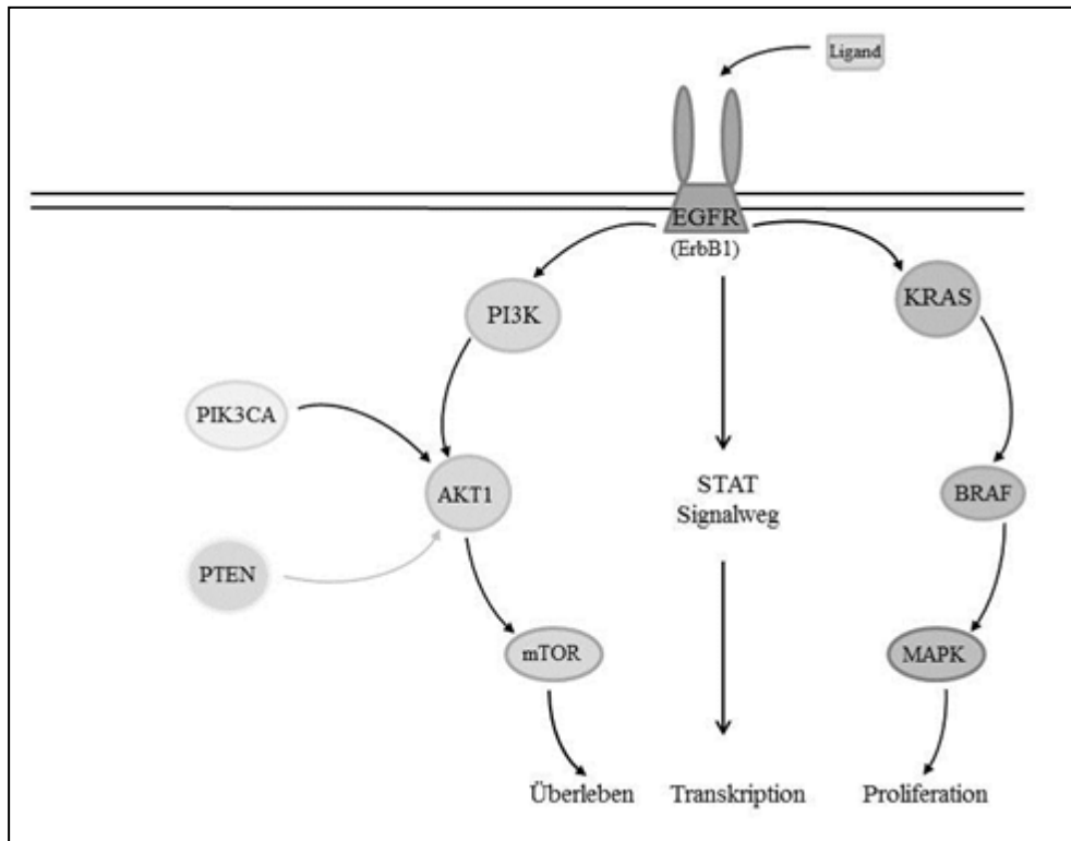
Abbildung 1: Signaltransduktionskaskade des EGFR
